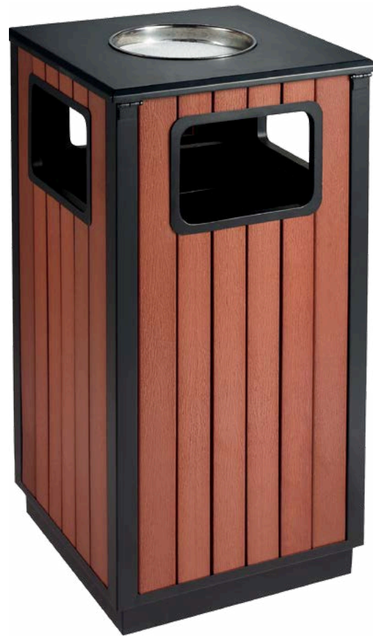
► MJR9494L SIZE: L450×W450×H850mm
